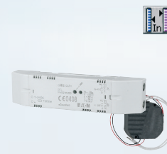
RF Analogové vstupy dvojité 0/10 V, 0-20 mA, 4-20 mA, PT1000 umožňují měření vlhkosti, teploty, intenzity osvětlení, kvality vzduchu - měření venkovní teploty, podlahové teploty, technologických teplot topení, chlazení, TUV
